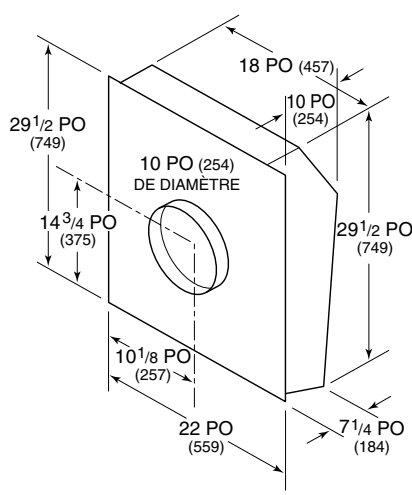
Ventilateur à distance de 1 200 pi³/min
