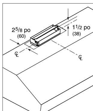
Évacuation verticale
