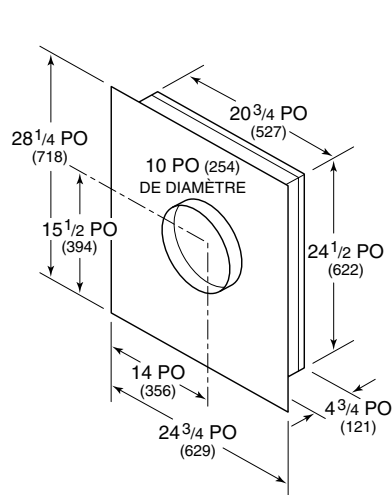
Ventilateur à distance de 600/900 pi³/min
