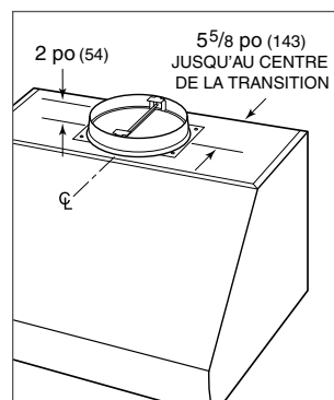
Évacuation verticale
